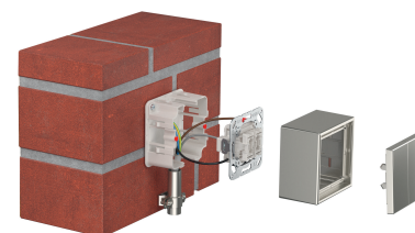
▲ Aufbau Lichtschalter bei Aufputz-Installation © JUNG
