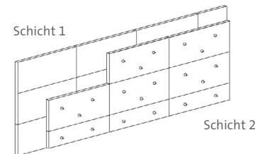
▲ Überdeckung von Wärmedämmplatten
