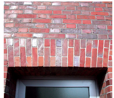
▲ Steindicker, scheitrechter Bogen
