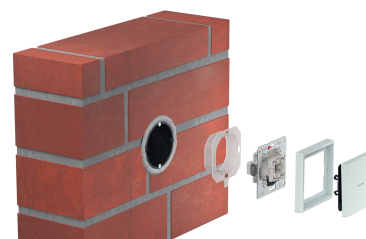
UNTERPUTZAUSFÜHRUNG
